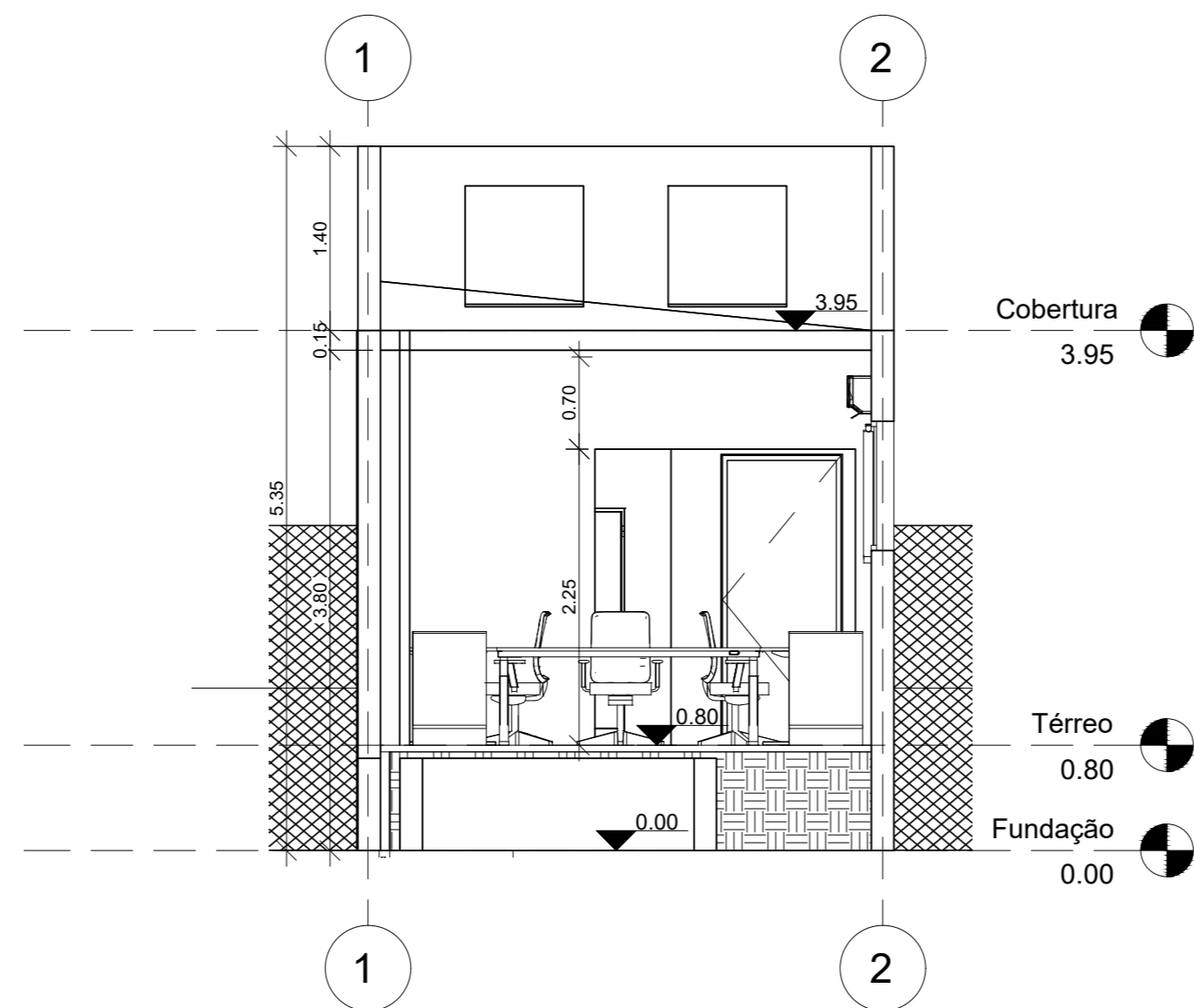
Corte BB 1 : 50
