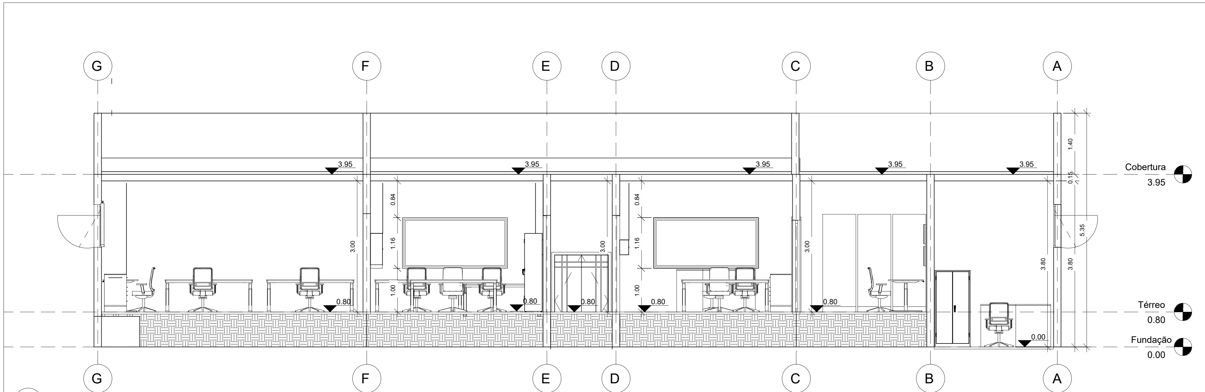
Corte AA 1 : 50
