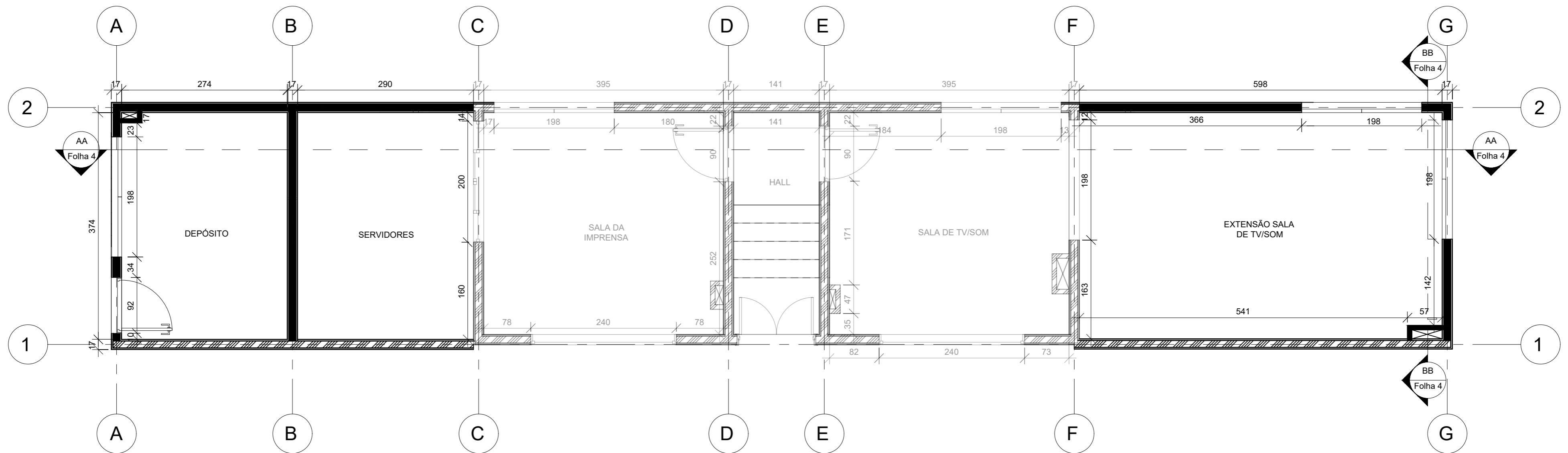
1 Térreo - EIXOS ESTRUTURAIS 1 : 50
